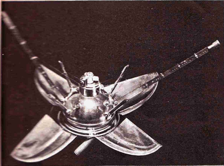
«Луна-13» получилась совсем как настоящая — четыре лепестка, две телекамеры, штыревые зеркала.
